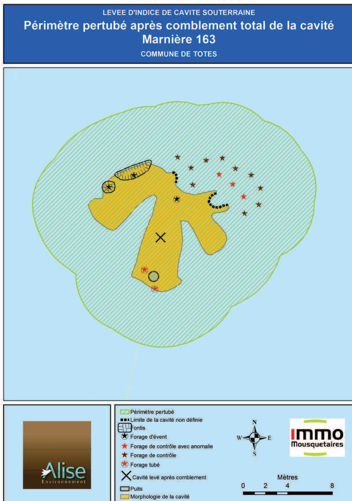
Figure 6 : Périmètre perturbé de la marnière 163
