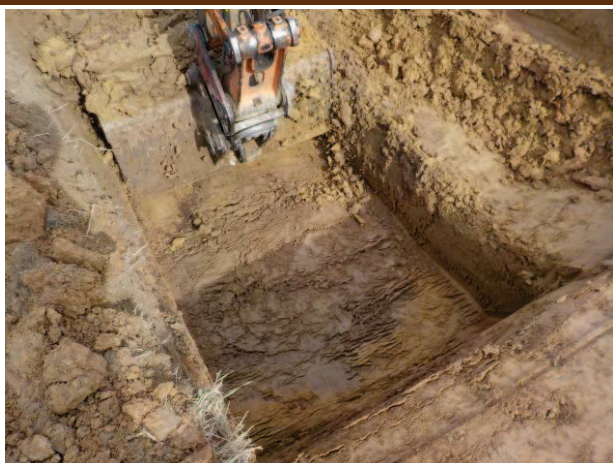
Photographie 13 : Poursuite de l'anomalie circulaire (ICS 241) et diminution de son diamètre (1,5m)
