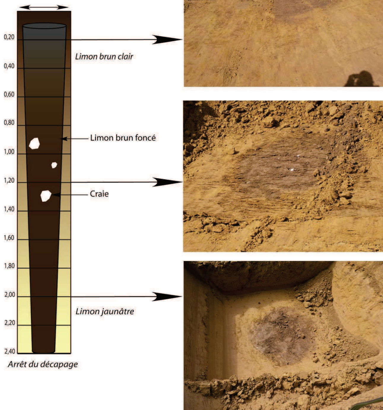
Figure 4 : Coupe synthétique des formations rencontrées (ICS 51)
