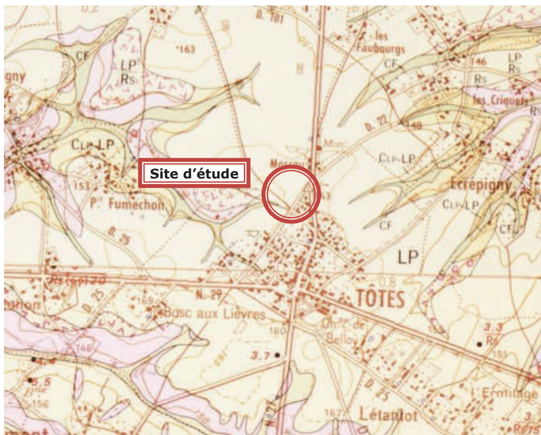
Figure 5 : Extrait issu de la carte géologique
