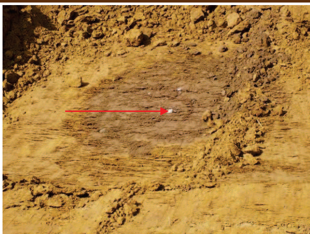
Photographie 17 : Poursuite de l'anomalie circulaire (ICS 51) à 1,2m, présence de craie
