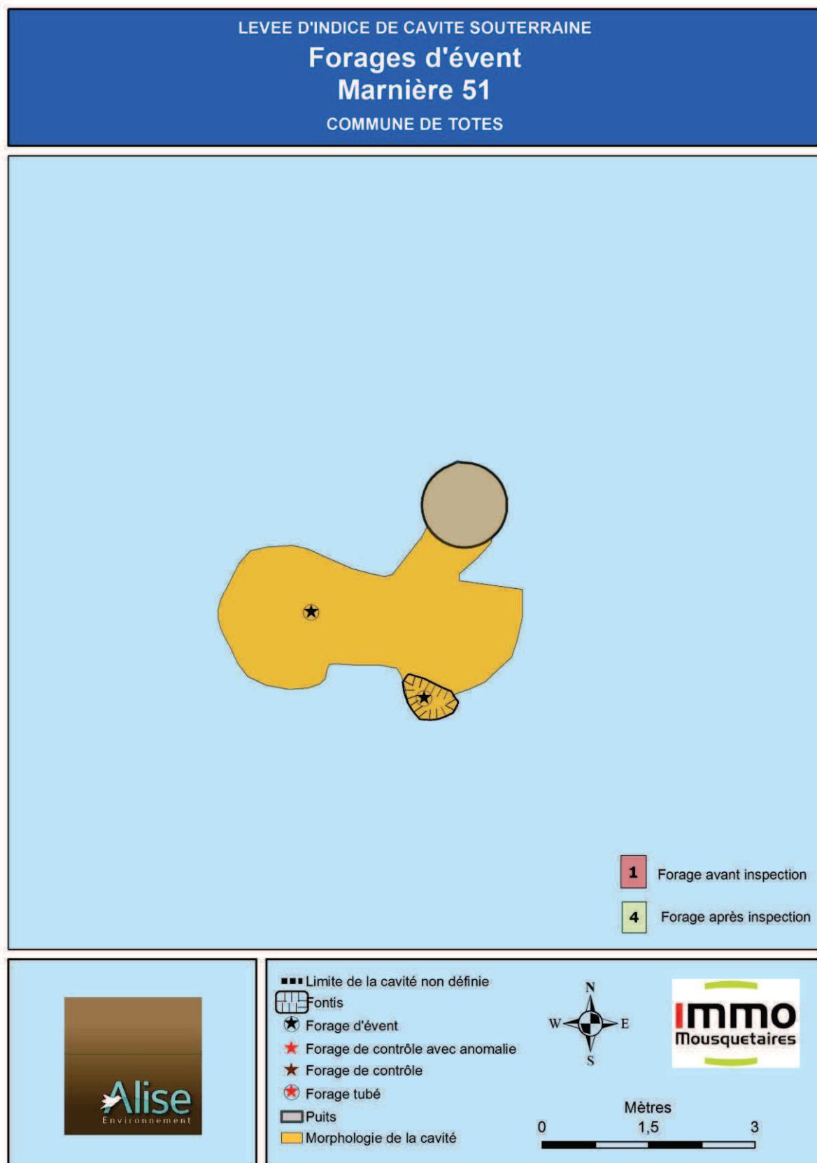
Figure 1 : Forages d'événements de la marnière 51
