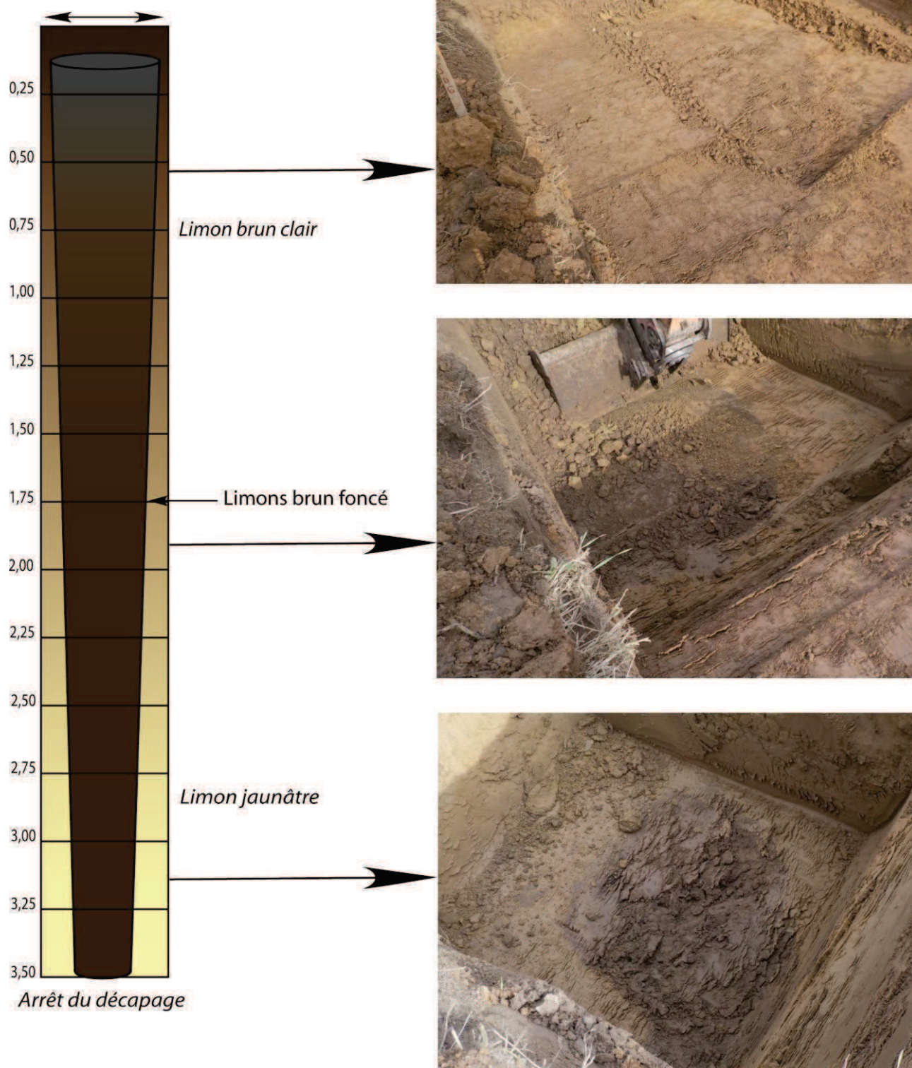
Figure 3 : Coupe synthétique des formations rencontrées (ICS 241)
