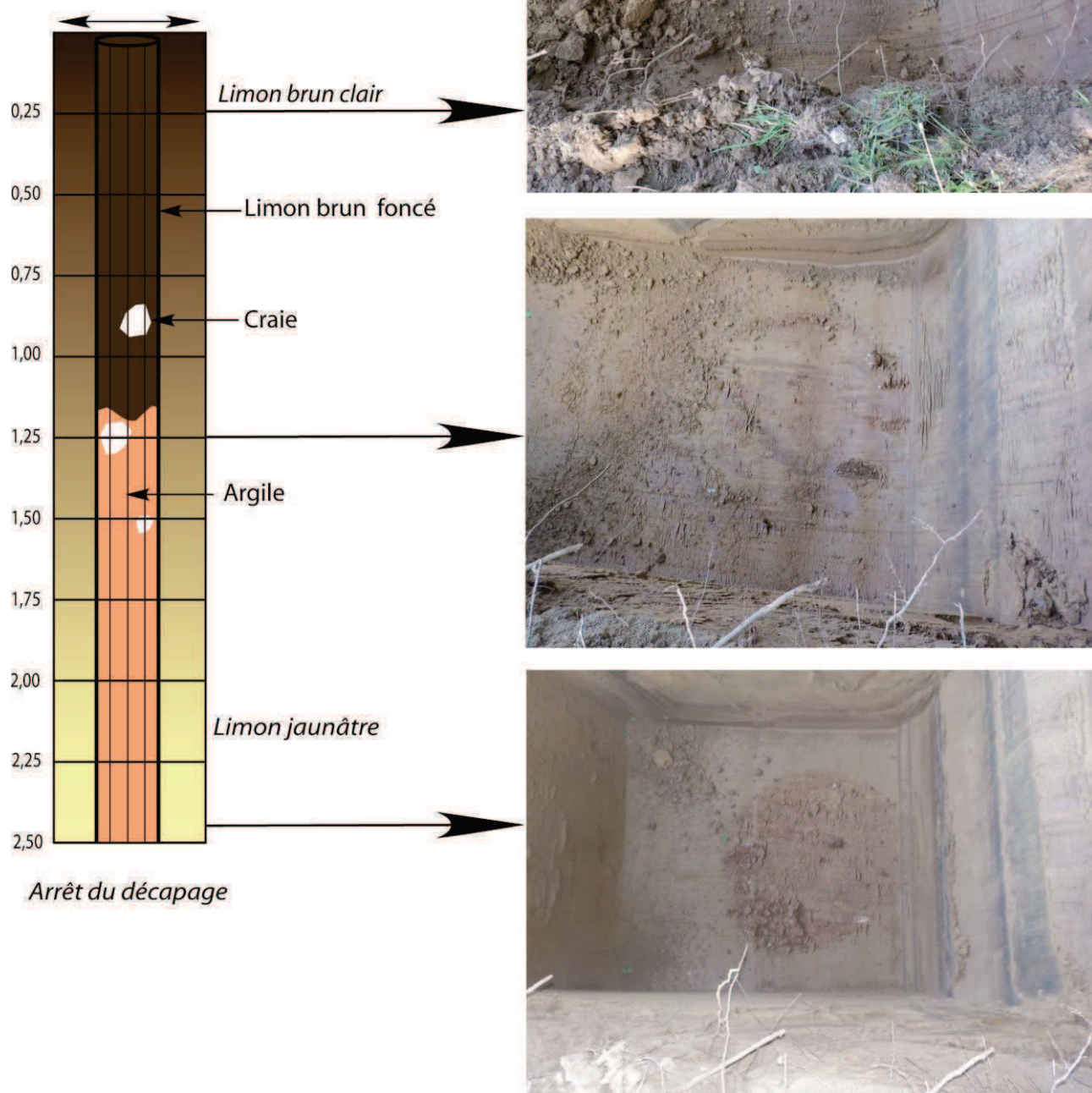
Figure 5 : Coupe synthétique des formations rencontrées (ICS 242)
