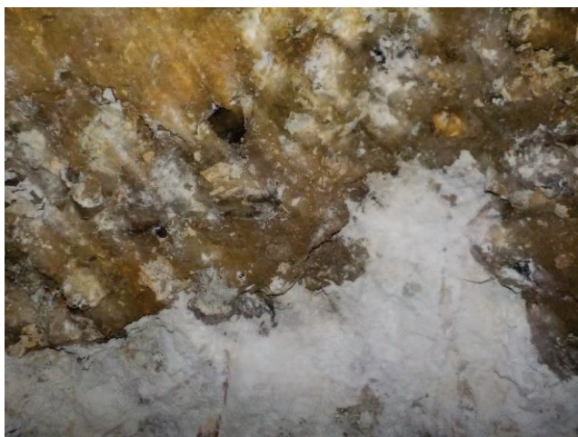
Photographie 3 : Puits recreusé le long d'un épi de marne et de l'autre côté, présence d'une racine d'argile à silex
