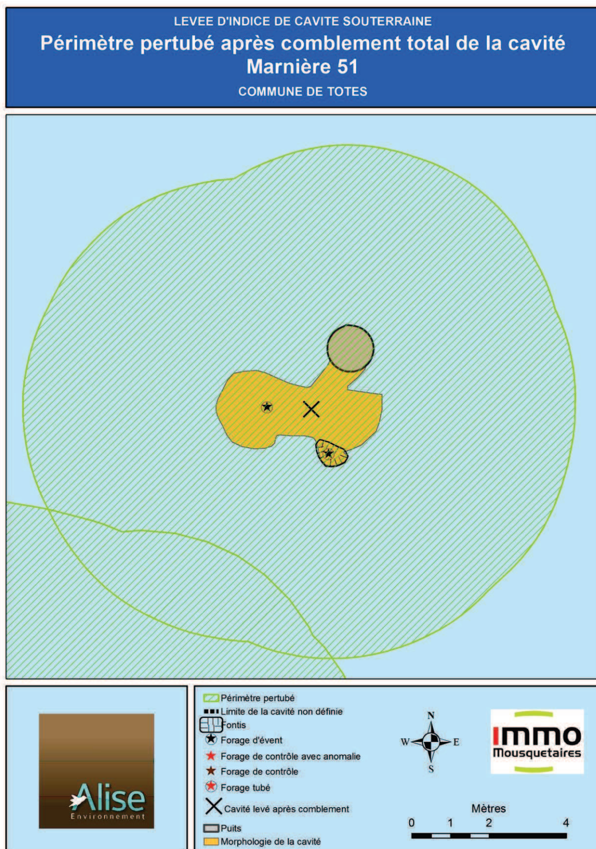
Figure 3 : Périmètre perturbé de la marnière 51
