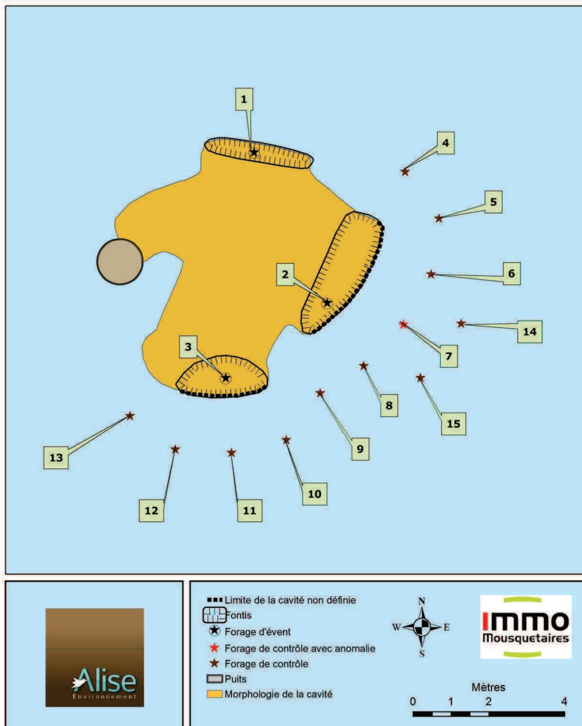
Figure 7 : Forages d'événements et forages de contrôle de la marnière 241
