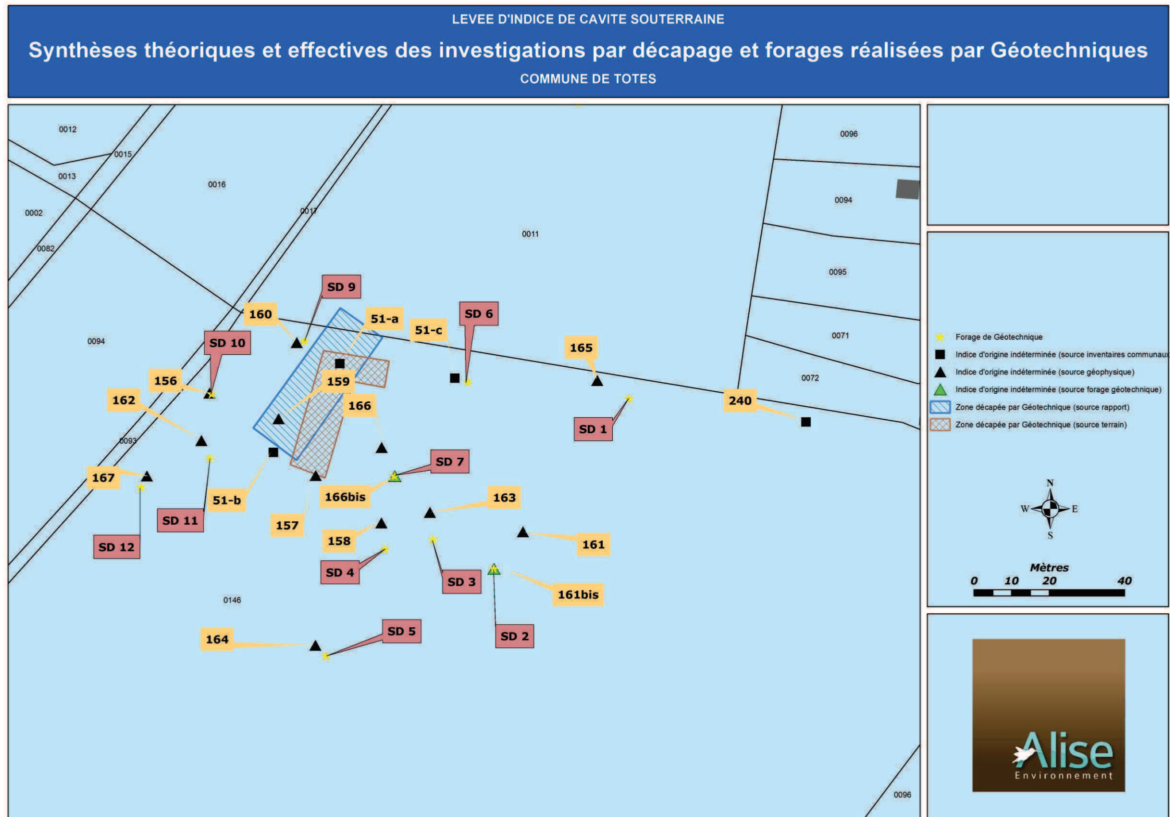
Figure 10 : Synthèses théoriques et effectives des investigations par décapage et forages réalisées par Géotechniques
