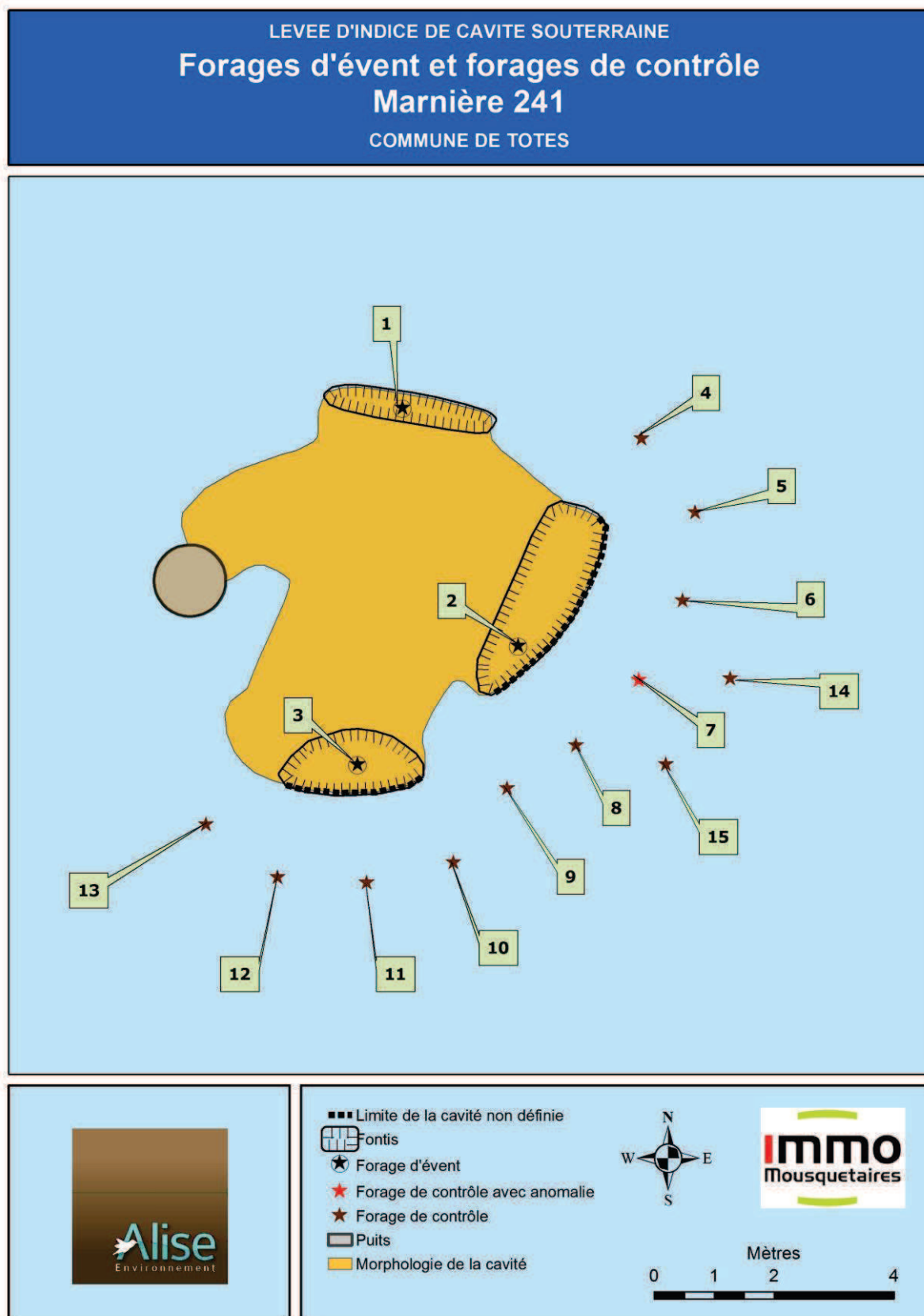
Figure 7 : Forages d'événements et forages de contrôle de la marnière 241
