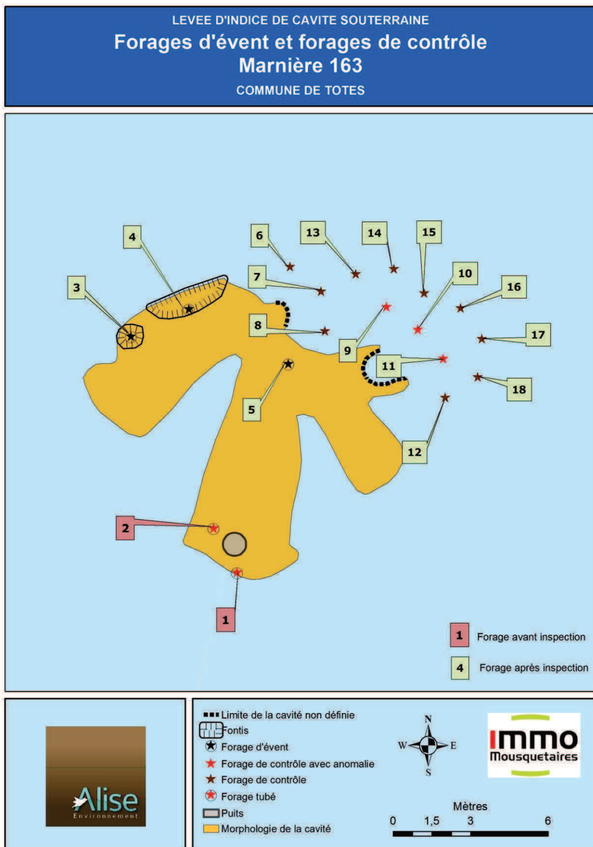
Figure 4 : Forages d'événements et forages de contrôle de la marnière 163
