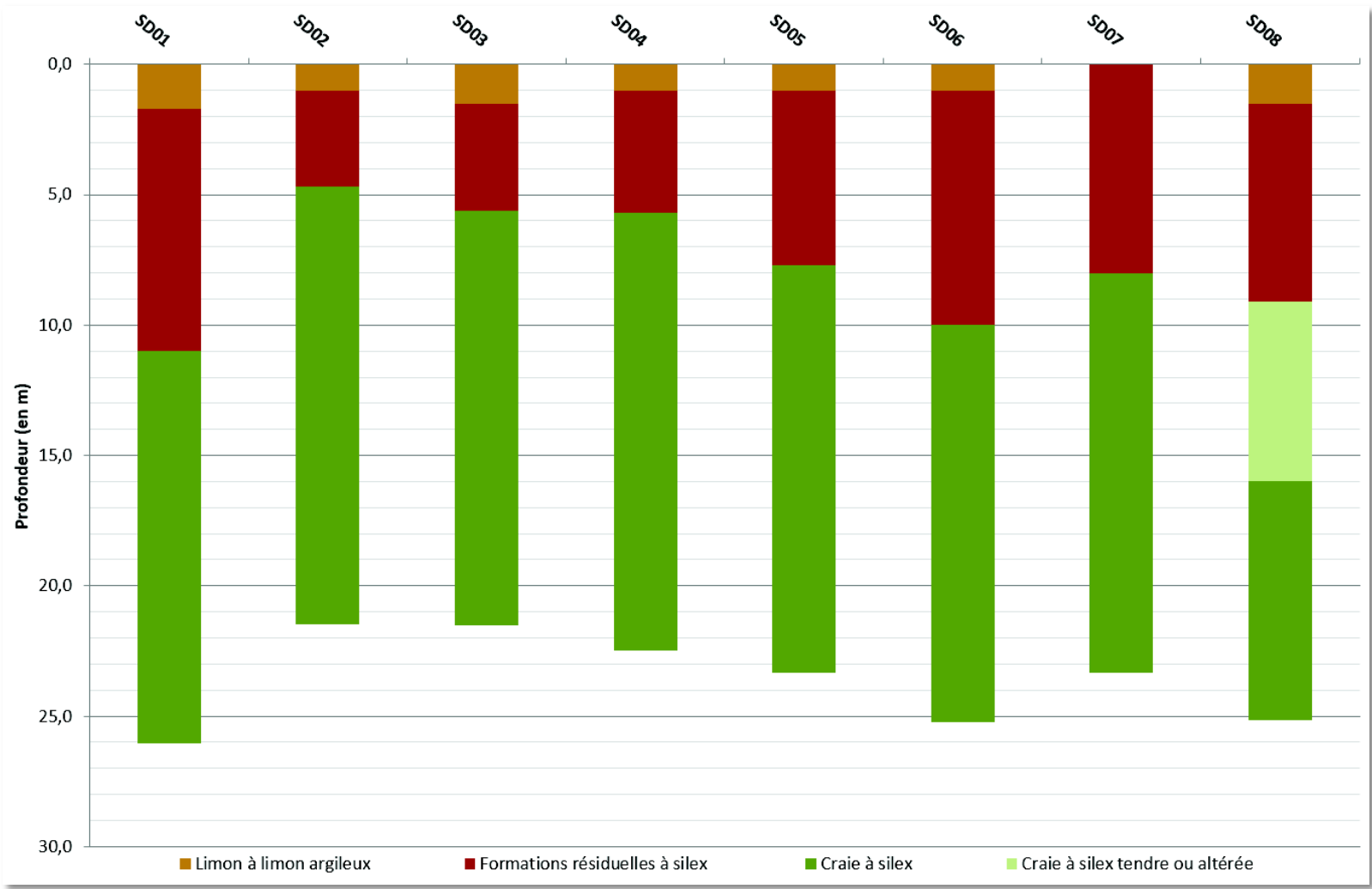
Schéma 6 : Synthèse lithologique établie à partir des sondages destructifs profonds
