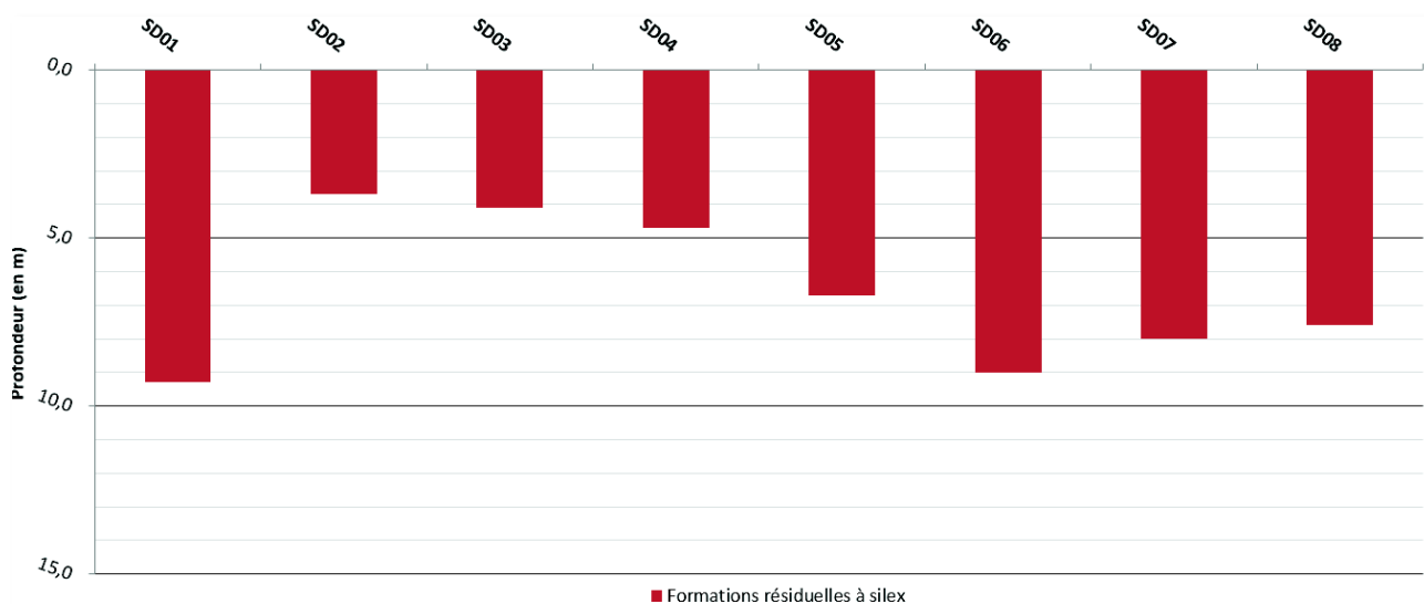
Graphique 2 : Variation des formations résiduelles à silex
