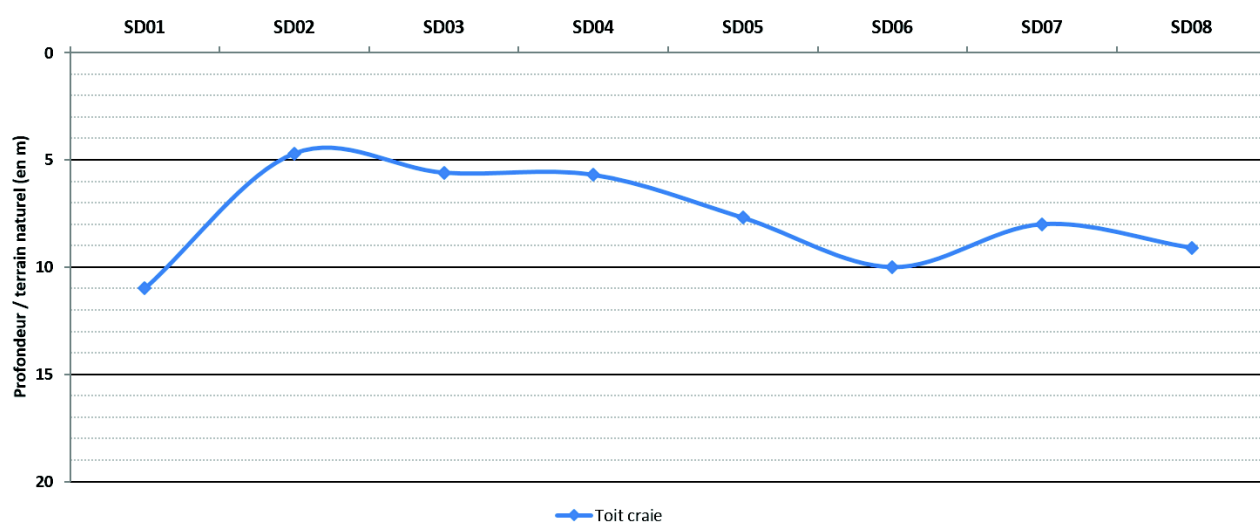
Graphique 3 : Variation de la profondeur du toit de la craie
