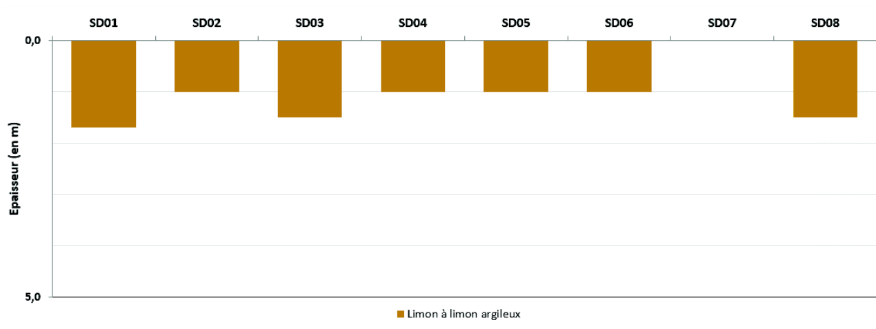
Graphique 1 : Variation d'épaisseur des formations limono-argileuses
