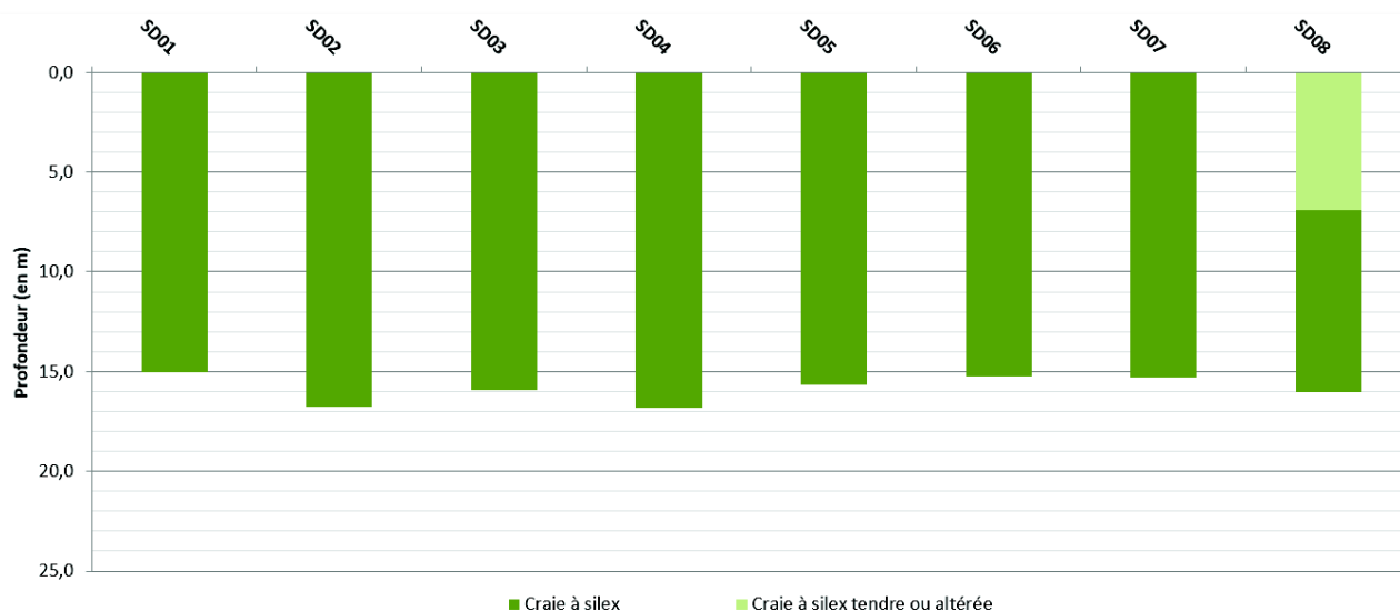
Graphique 4 : Variation d'épaisseur des formations crayeuses
