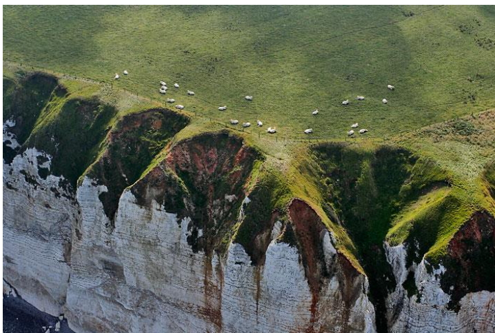
Vue aérienne de la falaise côtière on notera le "festonnage" lié à la succession de points durs (pinacles de craie) et de racines remplies de matériaux résiduels moins compacts
