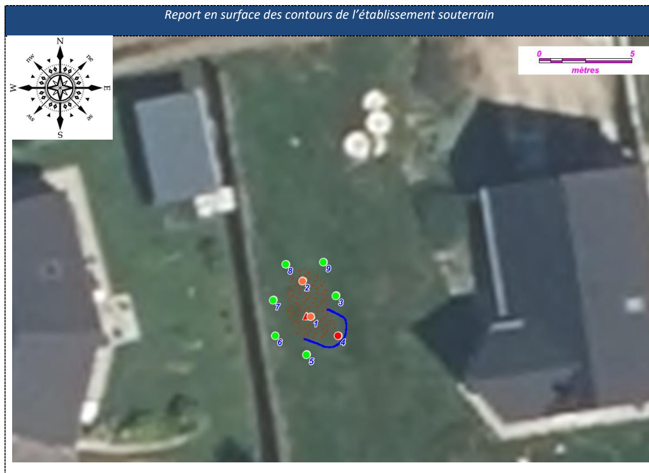
Schéma 11 : Report en surface des parties reconnues de la marnière souterraine à partir de SD4
