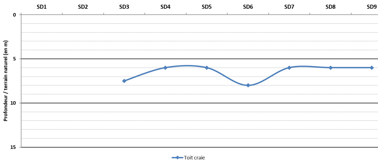
Schéma 8 : Profondeur du toit de la craie rencontré sur les sondages SD01 à SD09
