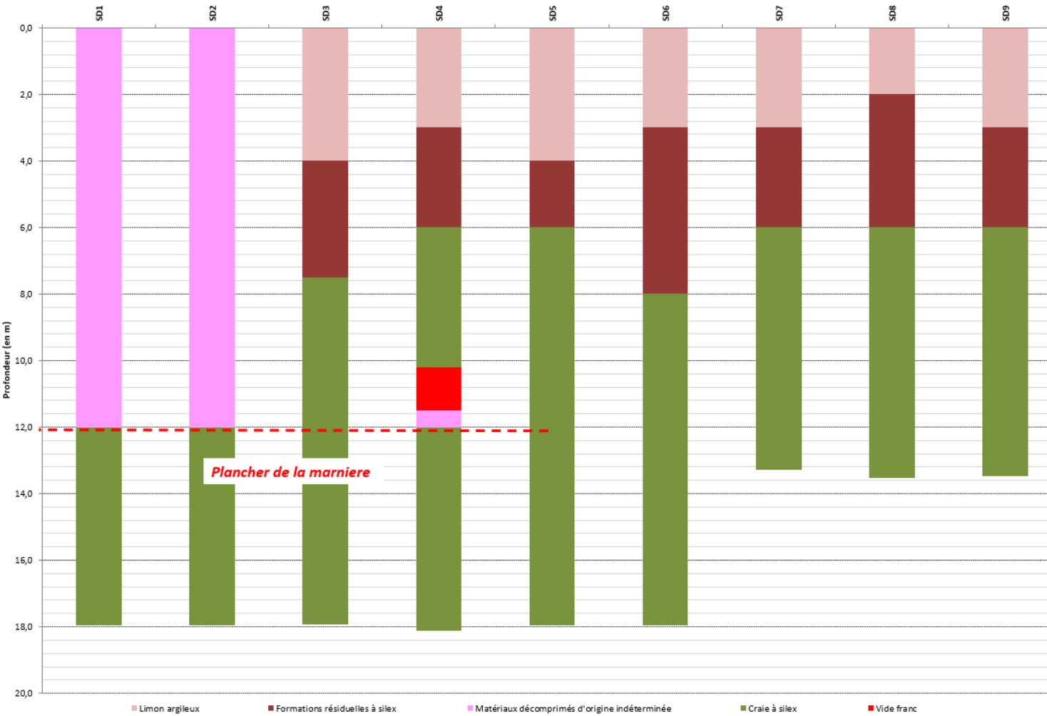
Schéma 9 : Synthèse lithologique des sondages 01 à 09
